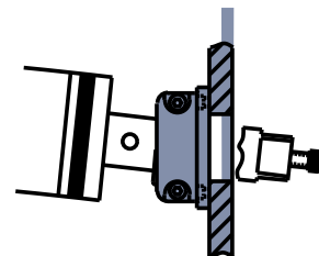
Brida (Interna)
